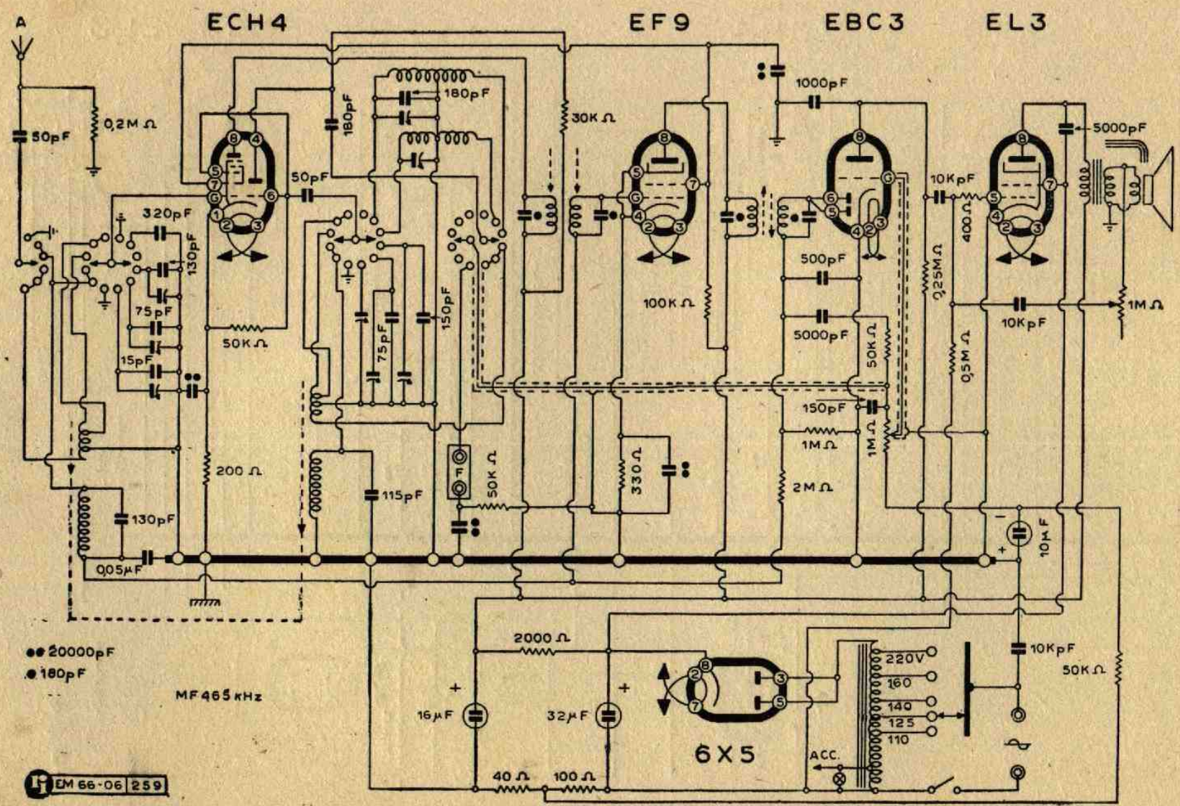
Lo schema elettrico del mod. R 951
